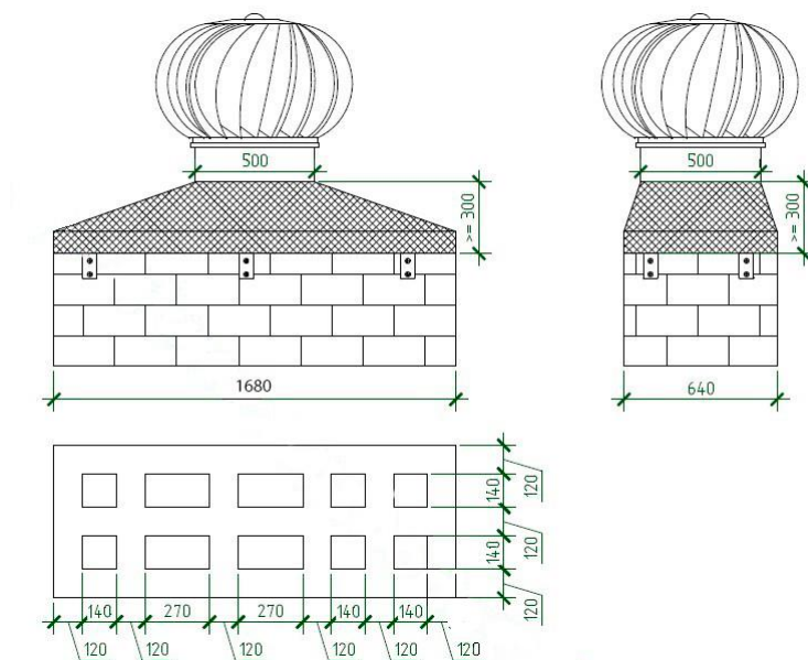
Рис. 2. Пример монтажа Турбодефлекторов через переход
