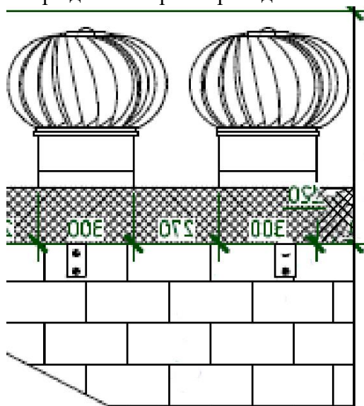
Рис. 1. Пример монтажа Турбодефлекторов через переход
