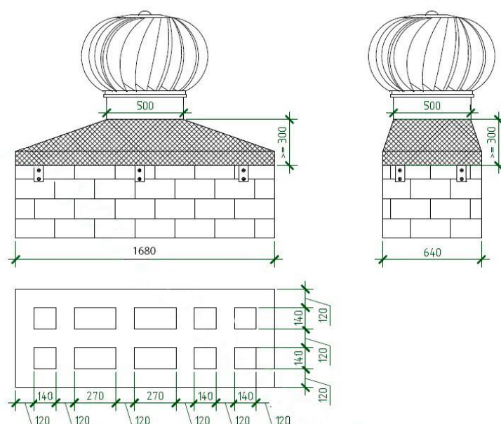
Рис. 4. Пример монтажа Турбодефлекторов через переход
